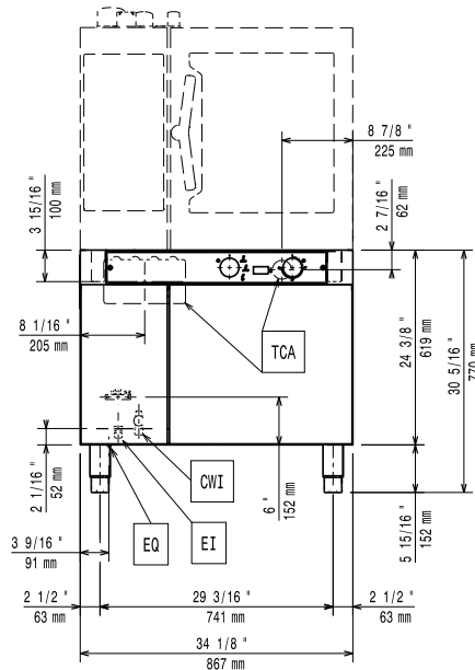
Front aanzicht
